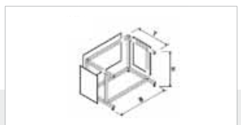
Sichtblenden für Pulttisch, Blech 1,5mm lackiert, Farbe: lichtgrau, mit Anschraubhalter Side panels desk type construction, Metal panels 1,5mm coated, colour lightgrey, with screw-on bracket Panneaux lateraux le modele pupitre, Tôle 1,5mm laque, couleur gris clair, avec équerre à panneaux
