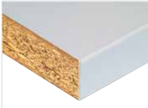
Spankernplatte melaminharzbeschichtet, 28 mm melamin-coated top 28 mm plateau mélaminé 28 mm
