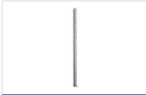
Multiwand-Tragsäule 30x60mm, für Plattenstärke 40mm. Bei 2m Länge werden 3 Tragsäulen benötigt. (And. Plattenstärken auf Anfrage) Upright 30x60mm for top 40mm. For length 2m 3 uprights are necessary. (For other worktops on demand) Montant 30x60mm pour plateau ép. 40mm. Pour une longueur de 2m 3 montants sont indispensables. (Pour d'autres plateaux sur demande)
