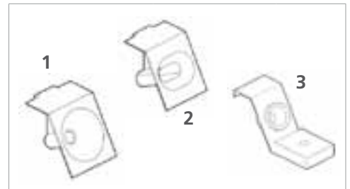
Werkzeughalter, 1: Halter f. Schraubendreher, 2: Halter für Zange, 3: Halter f. LötKolben Tool holder, 1: holder for screwdrivers, 2: holder for pliers, 3: holder for soldering irons Porte-outil, 1: support pour tournevis, 2: support pour pinces, 3: support pour fer à souder
