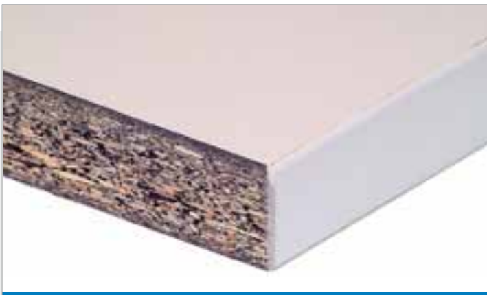
EGB-leitfähige Arbeitsplatte - Geeignet für alle elektrostatisch gefährdeten Bereiche, Oberfläche RAL 7035 ESD anti-static worktop for all electronic areas RAL 7035 / Plateau DCE anti-statique pour toutes les zones sensibles, RAL 7035
