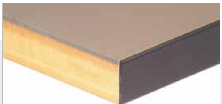
MDF-Platte mit robustem, strapazierfähigem Kunststoffbelag 2,5mm (Trovidur), 4-seitig ABS Umleimer - Schwer entflammbare Oberfläche, beständig gegen Salzlösungen, Säuren und Alkalien Worktop with 2,5mm high grade industrial linoleum surface TROVIDUR, edges anti-shock, nearly unflammmable and resistant against salt, acids and alkaline solutions Plateau robuste, recouvert d'un linoléum de 2,5mm, les bords antichoc, difficilement inflammable et résistant aux acides et solutions alcalines
