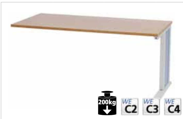
Anbautisch rechts, mit Getriebe für Kurbelverstellung und elektrischer Höhenverstellung, Platte Multiplex 25mm add-on module RHS, with gears (for crank, 1 or 2 motors) top multiply 25 mm Module addit. à droite, avec transmission (pour manivelle, 1 ou 2 moteurs) plateau multiplis 25 mm
